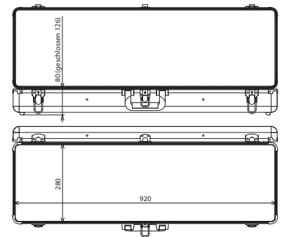
Maßbild KKL 92 28 12
