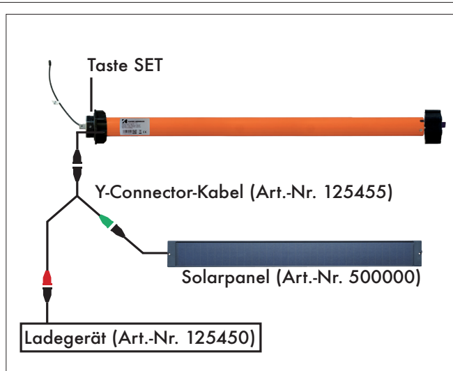
Abb.1: Anschlussbeispiel Junior Easyline - KB
