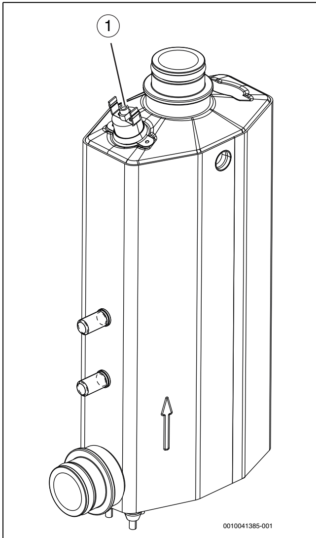
Bild 43 Elektrischer Zuheizer
