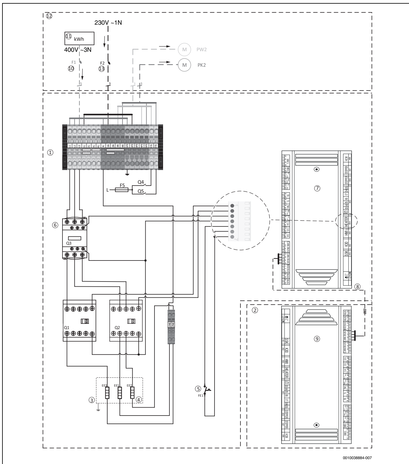
Bild 50 Spannungsversorgung Inneneinheit
