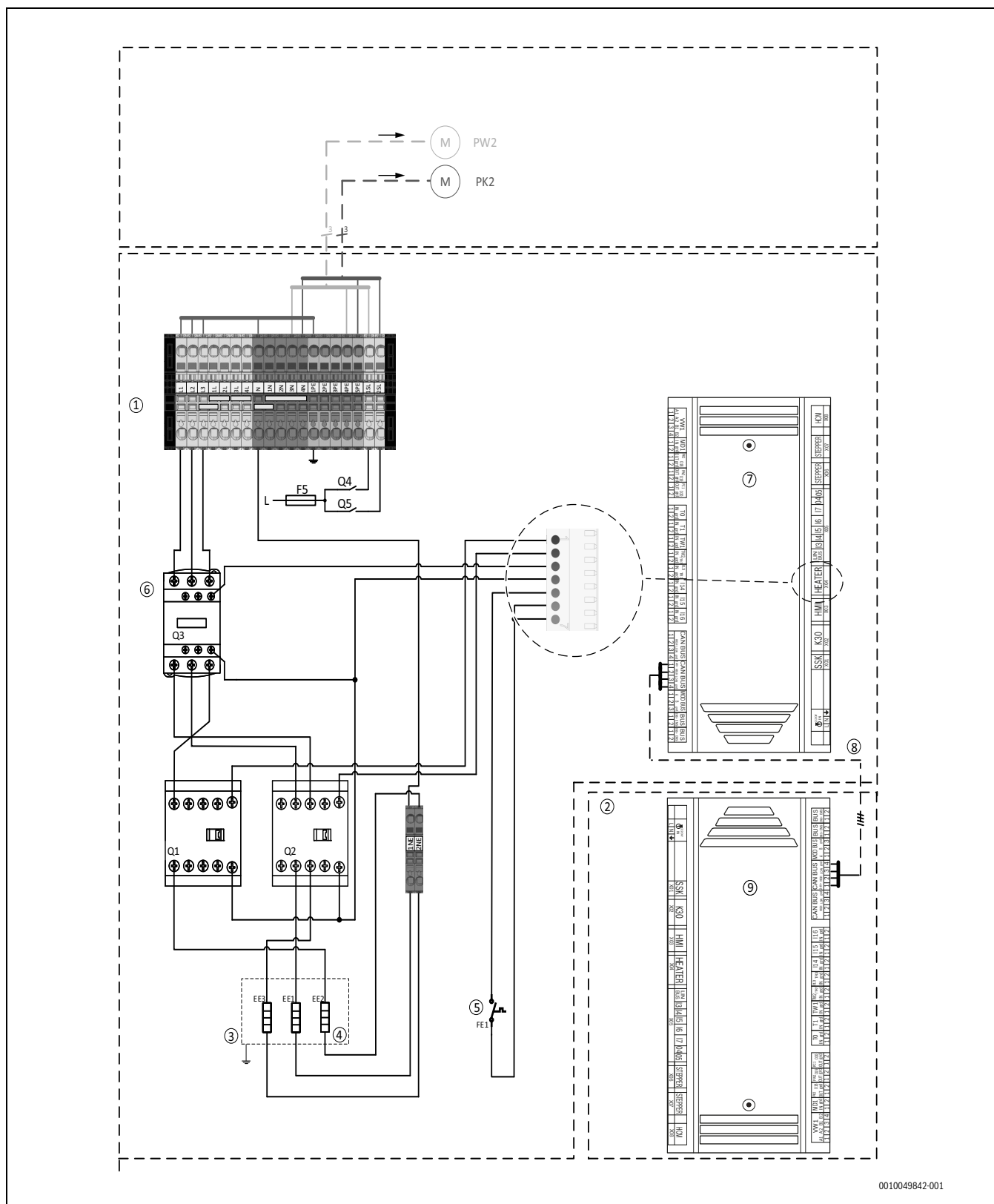
Bild 51 Spannungsversorgung Inneneinheit
