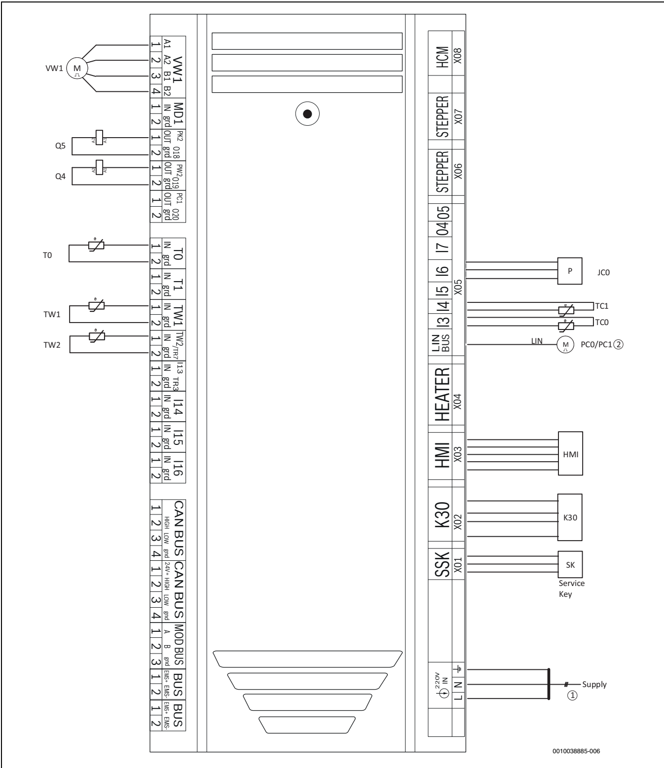
Bild 49 Schaltplan XCU-THH (XCU HY)-Modul
