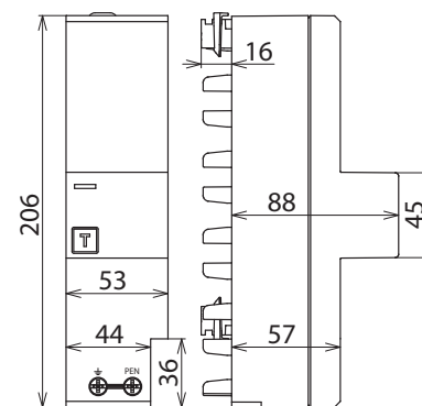
Maßbild DV ZP TNC 255
