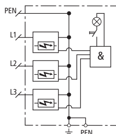
Prinzipschaltbild DV ZP TNC 255
