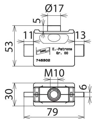
Maßbild EP NH00 TI M10
