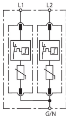
Prinzipialschaltbild DG MU SP 480 3W+G
