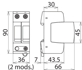
Maßbild DG MU SP 480 3W+G
