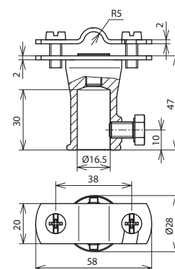
Maßbild LH 7.10 BB16 V2A ZG
