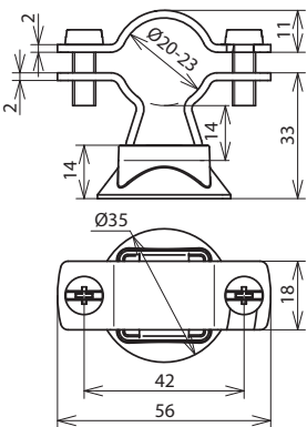
Maßbild LH ZS 20 23 KS H10 V2A
