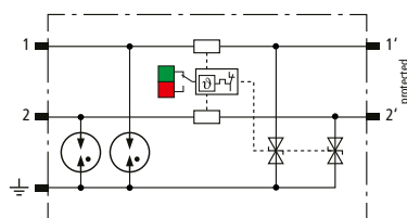
Prinzipschaltbild BCO MOD ML2 BE 48
