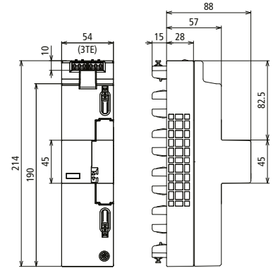
Maßbild DSH ZP 2 LSG TT 255
