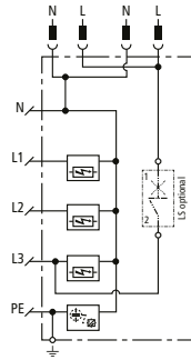
Prinzipschaltbild DSH ZP 2 LSG TT 255
