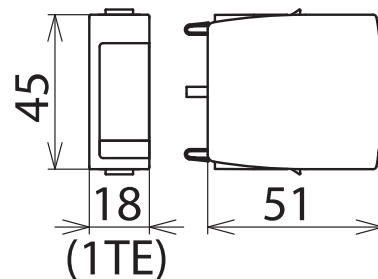
Maßbild DG MOD 150
