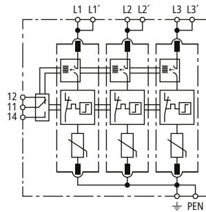
Prinzipschaltbild DG MP TNC ACI 275 FM
