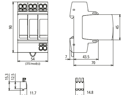
Maßbild DG MP TNC ACI 275 FM
