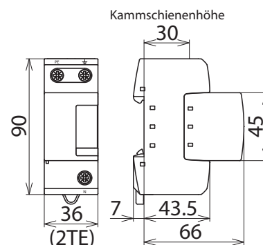
Maßbild DGP M 255
