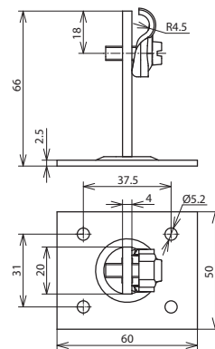
Maßbild DLH DQ 6.10 GP50X60 STTZN
