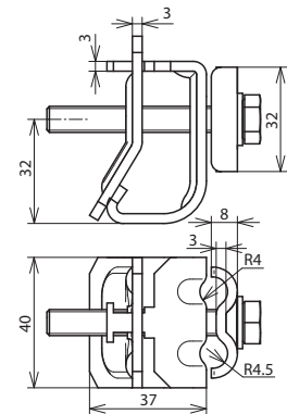
Maßbild DRK DUL 8.10 W16.22 EST AL
