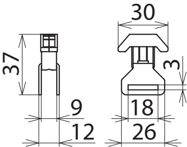
Maßbild AK 35 SN 18X3 GG
