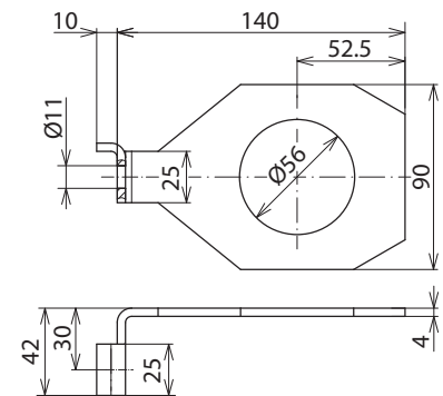
Maßbild AB EXFS IF1 W 56
