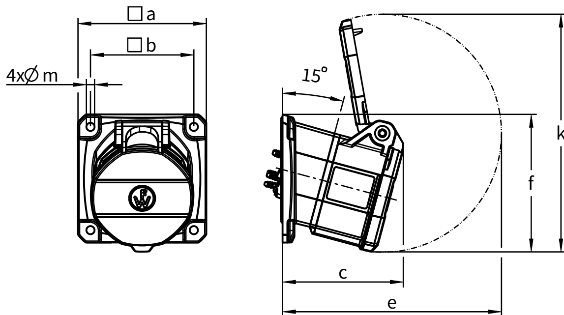
Montageausschnitt Mounting cutout
