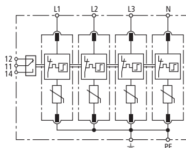
Prinzipialschaltbild DG M TNS 385 FM
