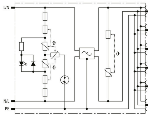
Prinzipschaltbild SFL PRO 6X 19"
