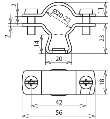
Maßbild LH ZS 20 23 GM6 V2A
