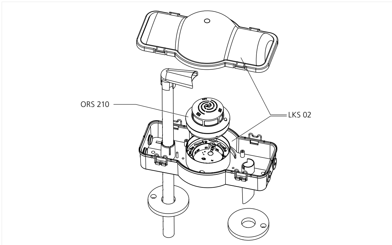
Abb. 1: Lüftungs-Rauchschalter-System LRS 01
