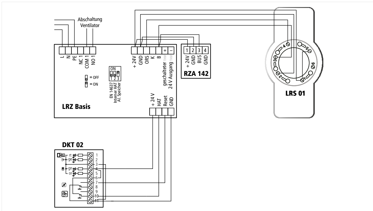
Abb. 6: Anschaltung LRZ Basis ohne Leitungsüberwachung
