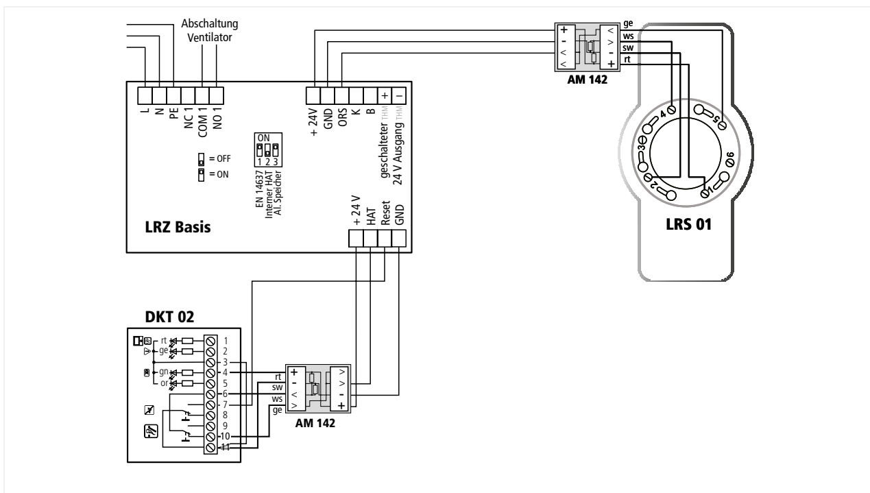
Abb. 7: Anschaltung LRZ Basis mit Leitungsüberwachung
