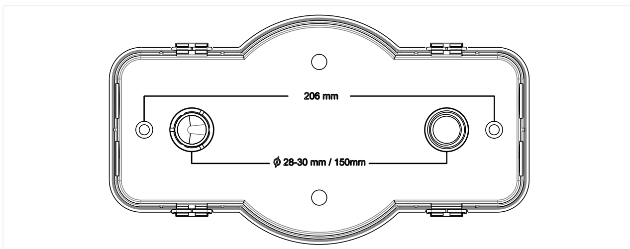
Abb. 5: Bohrmaße
