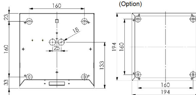
Bohrpläne:
