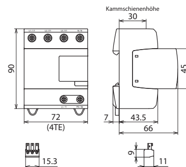
Maßbild DV M2 TT 255 FM
