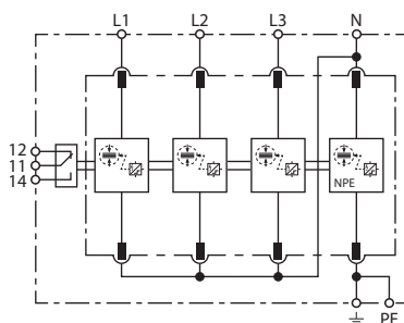
Prinzip Schaltbild DV M2 TT 255 FM
