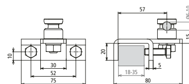
Maßbild AK 6.10 KSV FER W KBF18 35 V2A
