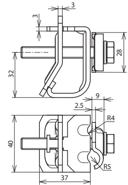
Maßbild DRK DUL 8.10 W16.22 EST STTZN
