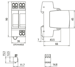
Maßbild DG MP TN 150 FM
