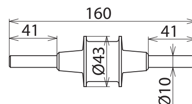
Maßbild KFSU
