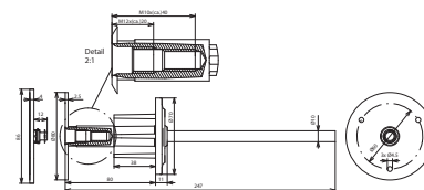
Maßbild EFPM M10 12 V4A WS L245 VP
