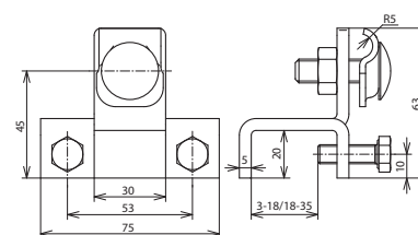
Maßbild AK 6.10 KB S KBF3 18 STTZN
