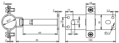
Maßbild LH ZS 27 EX W85 BP V2A
