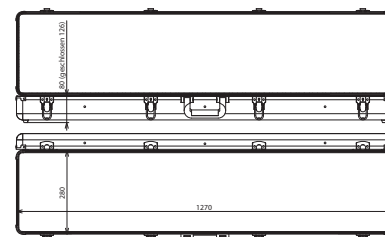
Maßbild KKL 127 28 12
