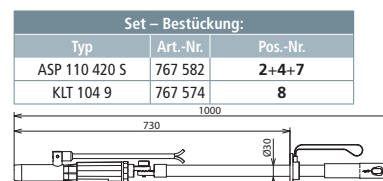
Maßbild ASP 110 420 S
