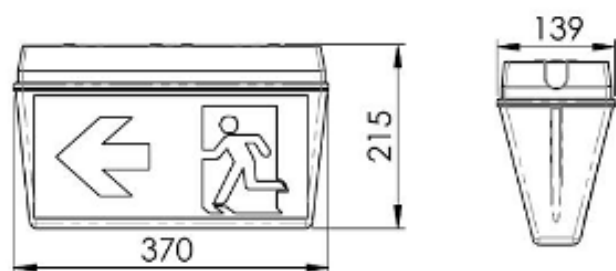
Maßzeichnung | dimensional drawing
