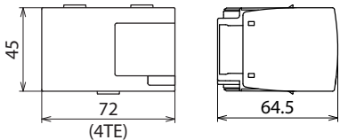
Maßbild DV MOD TNC 255
