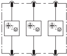
Prinzipschaltbild DV MOD TNC 255
