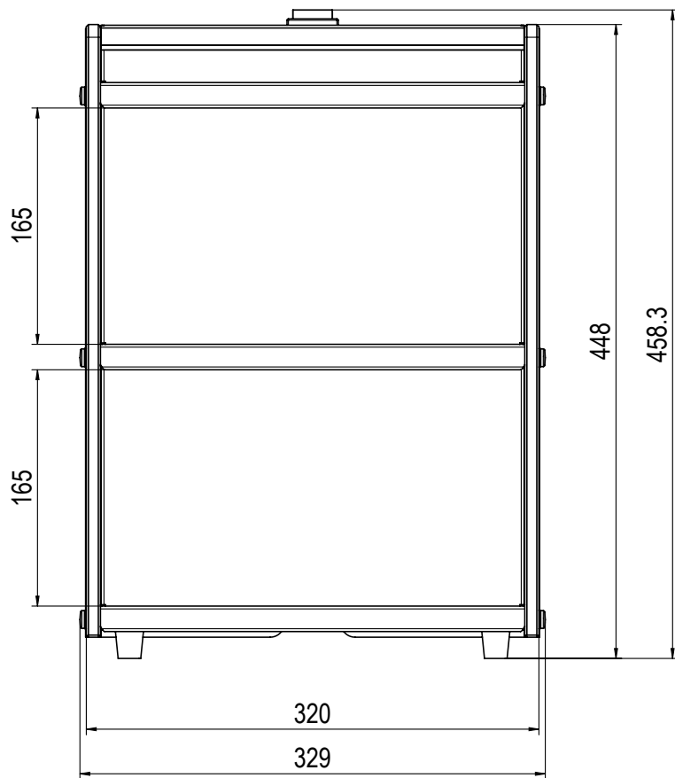
Aufriss
