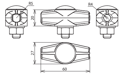
Maßbild ESTK 8.10 ZG
