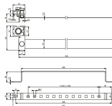
Maßbild BRS 16.168 ES 12AP V2A SET
