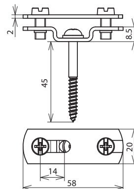
Maßbild FBH ZS 30 B6.5X16 HS5X50 V2A
