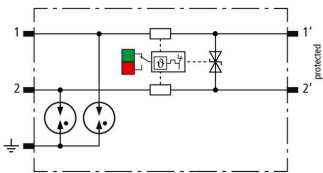
Prinzipschaltbild BCO CL2 BD 24
