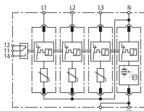
Prinzipialschaltbild DG M H TT 275 FM
