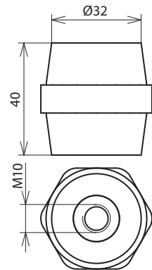
Maßbild IS PAS M10
