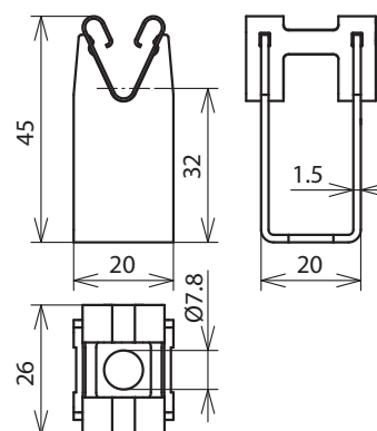
Maßbild LH DG 8 H32 B7.8 CU
