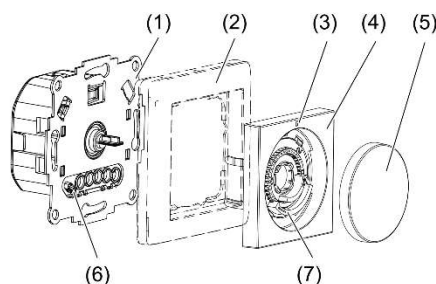
Bild 1: Geräteaufbau
