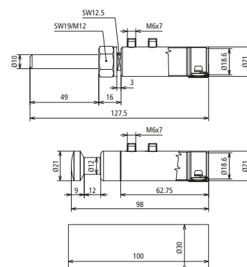
Maßbild HVI LI PL ASS RIV KF V2A
