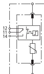
Prinzip Schaltbild DG S WE 600 FM
