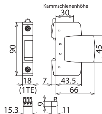
Maßbild DG S WE 600 FM
