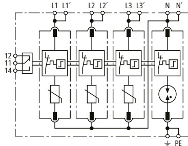
Prinzipschaltbild DG MD TT 385 FM
