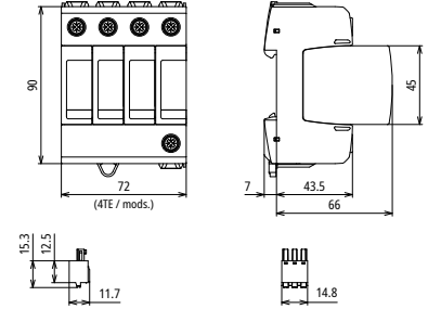
Maßbild DG MD TT 385 FM
