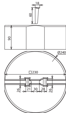
Maßbild BES 8.5KG KT10 16 D240 SET
