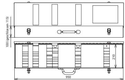
Maßbild SKL 95 21 10
