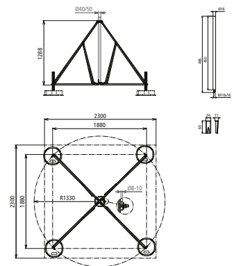
Maßbild VBS KB D50 RA1330 V2A
